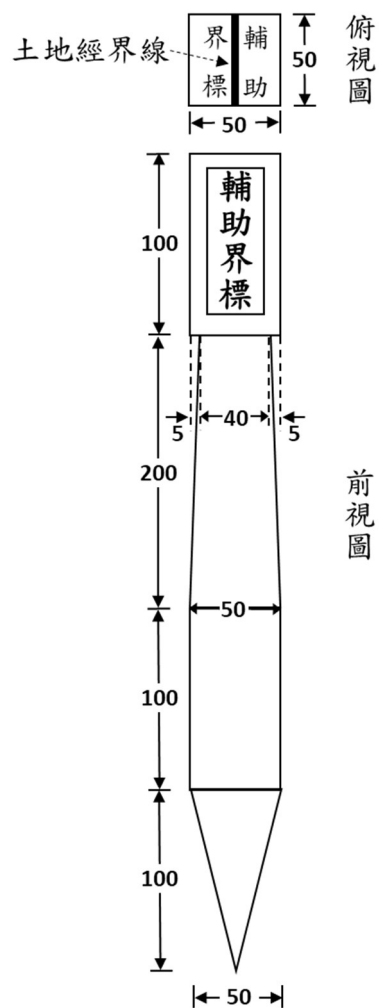
塑膠界標（輔助界標）
