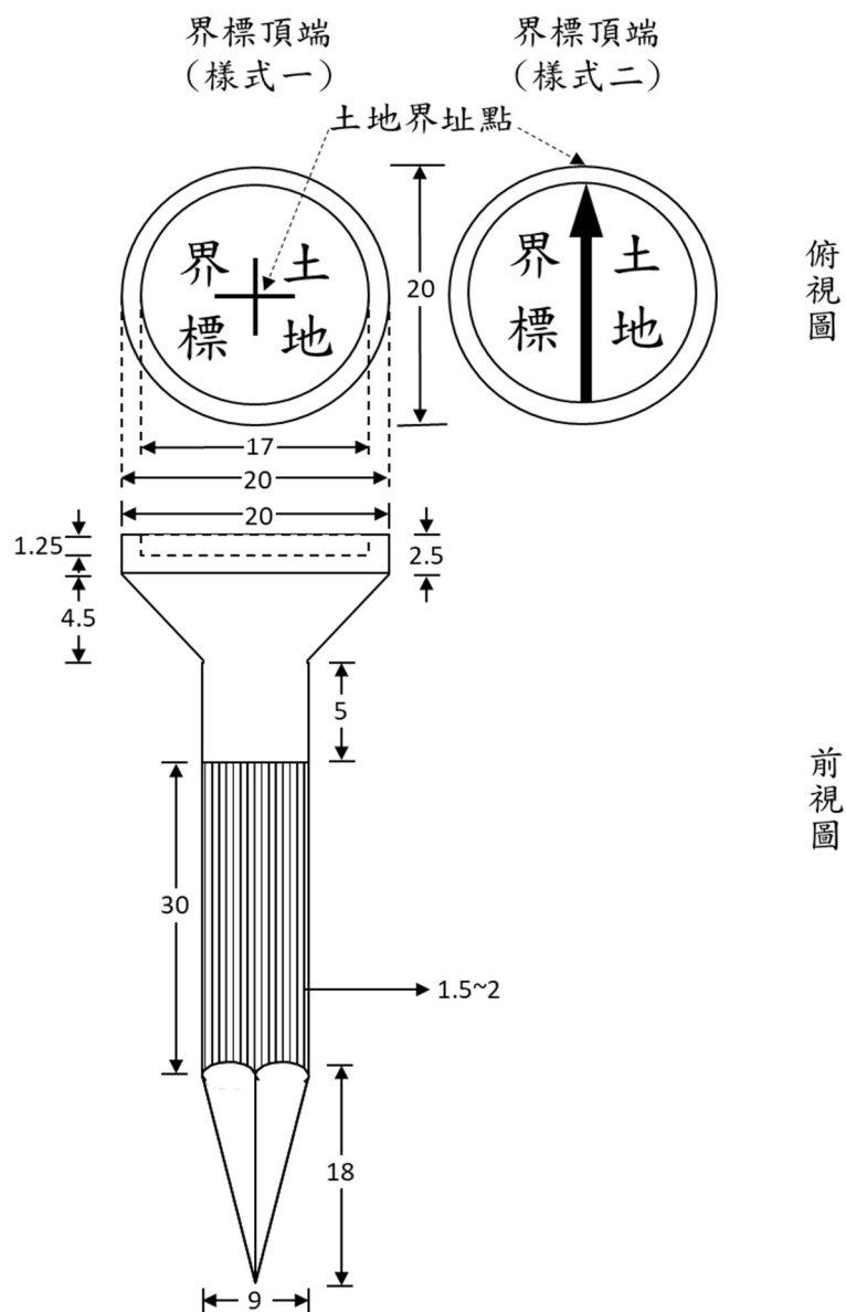
鋼釘界標（土地界標）
