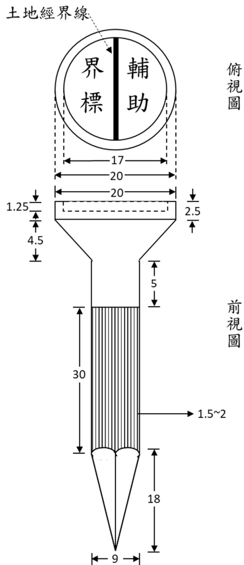
鋼釘界標（輔助界標）
